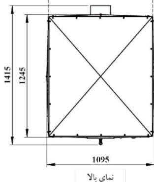
نمای بالا
