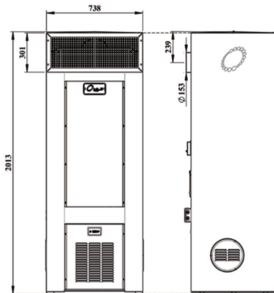
نمای روبرو
