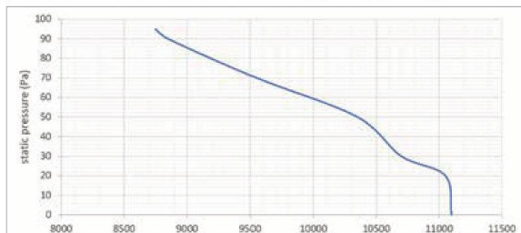
نمودار ۱ - نمودار هوادهی - افت فشار
