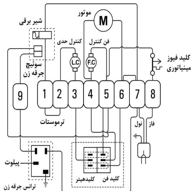
نقشه برق GH 625
