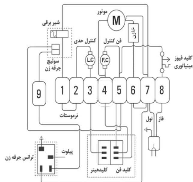
نقشه برق GH 640
