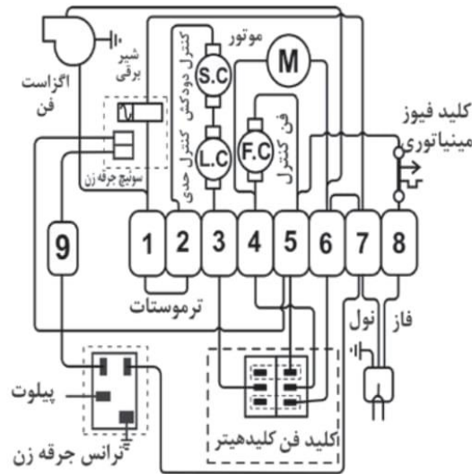
نقشه برق GH0625 sa
