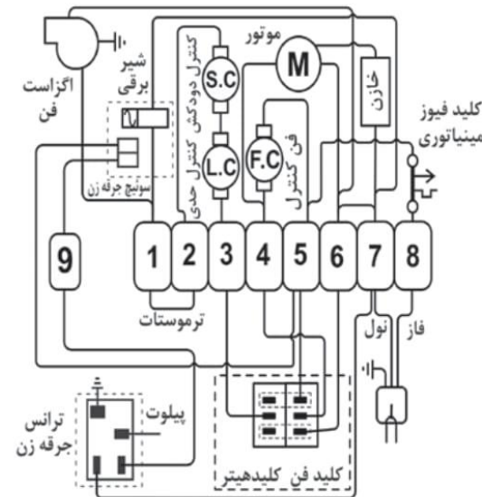
نقشه برق GH0640 sa
