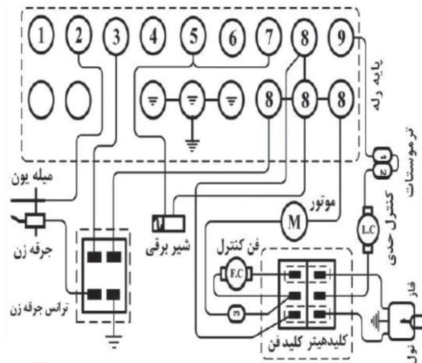
نقشه برق GH0640A-GH0625A
